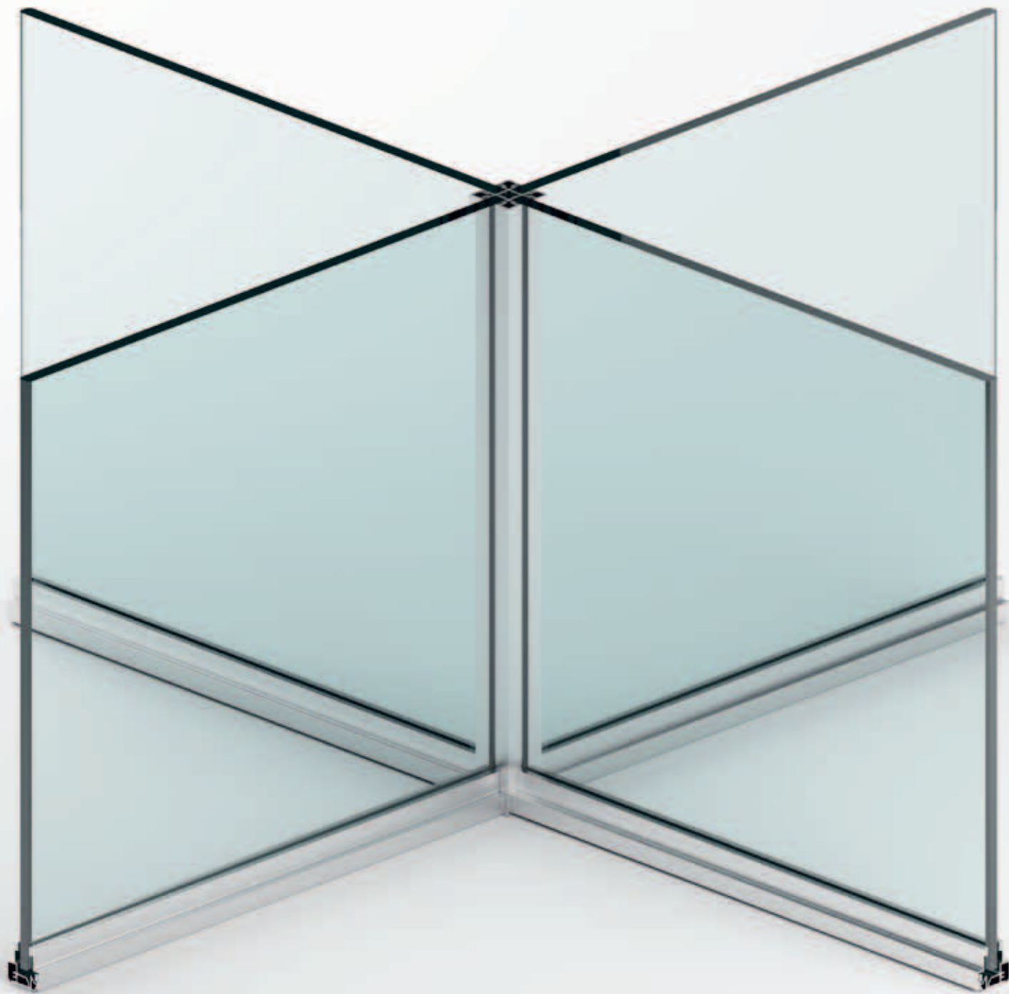
Connessione angolare 4 vie 90° 4-ways corner joint 90° 4 Wege Eckverbindung 90° Jonction angle 4 voies 90° Montante a 4 vías 90°
