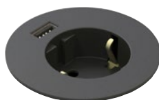
935-PM61 POWERDOT MIDI, ZWART 1 STROOM, 1 USB LADER (2.1 A) 1.7 M CONNECTIE (SCHUKO) VAST NIVEAU. HOOGTE 82 MM.
